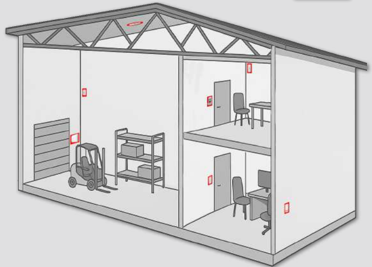
Pulsanti antipanico, rilevatori di movimento
